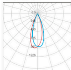
Narrow 26° 6W
